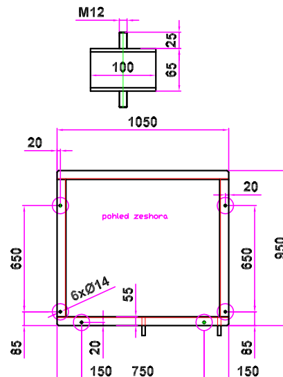
Silent bloky a rám GP300
